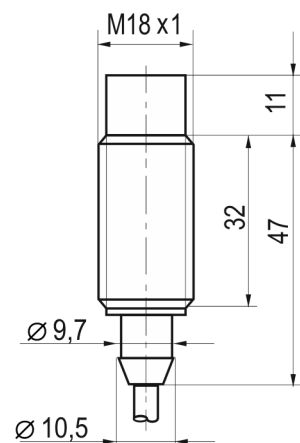
Габаритный чертеж
